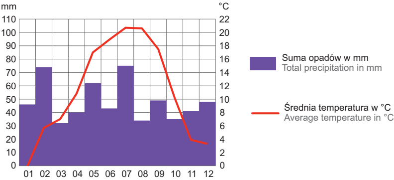
WYKRES 1. TEMPERATURY POWIETRZA I OPADY ATMOSFERYCZNE W STACJI METEOROLOGICZNEJ W TORUNIU W 2024 R. CHART 1. AIR TEMPERATURES AND ATMOSPHERIC PRECIPITATION IN METEROLOGICAL STATIONS IN TORUŃ IN 2024
